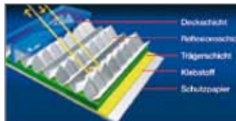
Reflexfolien-Aufbau RA3C Mikroprismentechnologie
