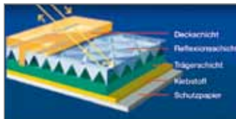
Reflexfolien-Aufbau RA2C Mikroprismentechnologie
