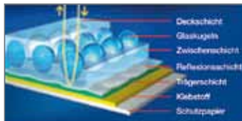
Reflexfolien-Aufbau RA1 Eingebundene Glasperlentechnologie
